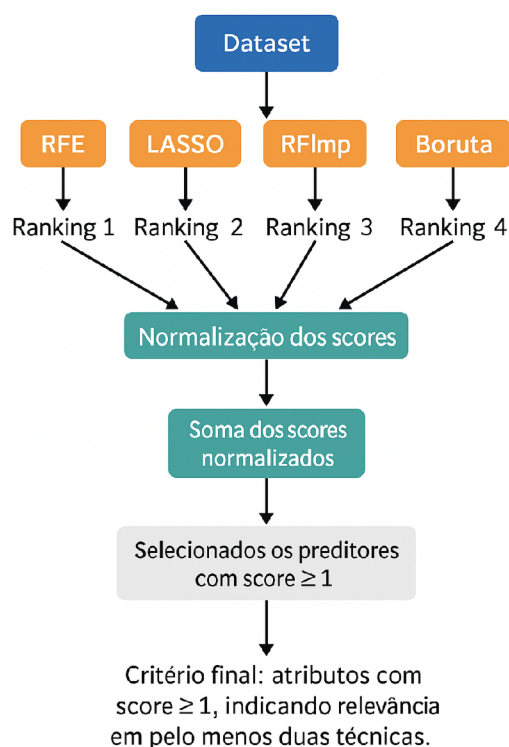
Figura 14: Fluxo de integração das técnicas de seleção de atributos.
