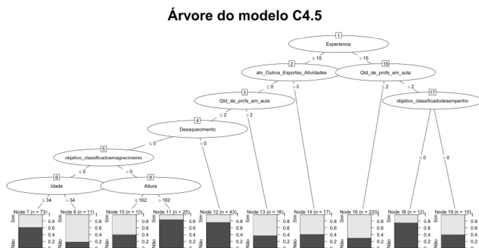
Figura 33: Árvore de decisão gerada pelo modelo C4.5 (J48) após tuning dos hiperparâmetros.
