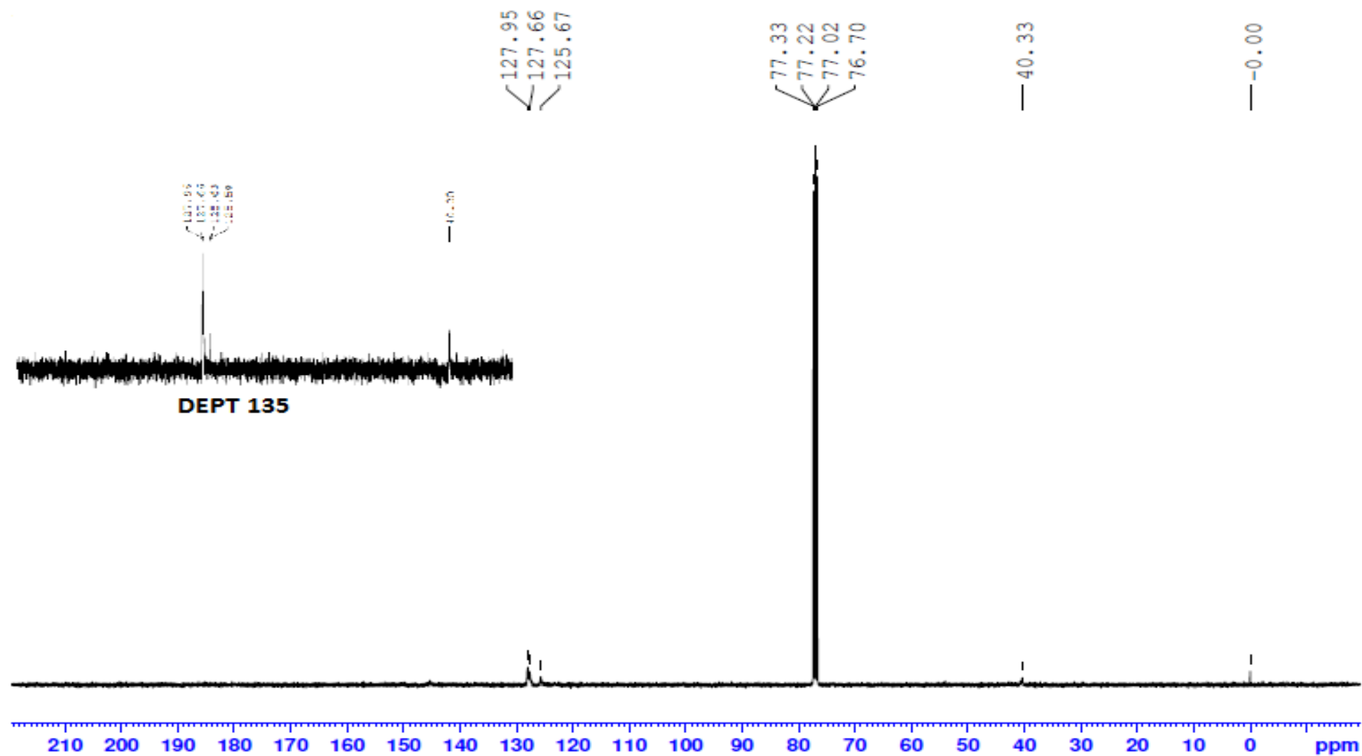
Figura 5. Espectro RMN ^{13}\text{C} e DEPT 135 do copolímero AA5, em \text{CDCl}_3
