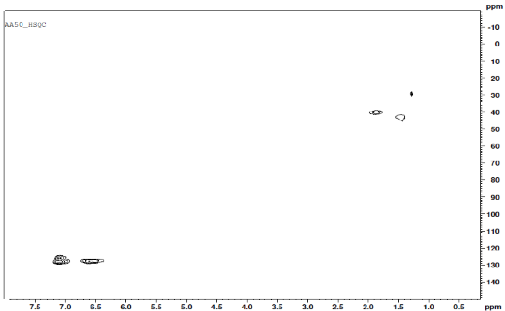
Figura 15. Espectro RMN HSQC do copolímero AA50, em \text{CDCl}_3
