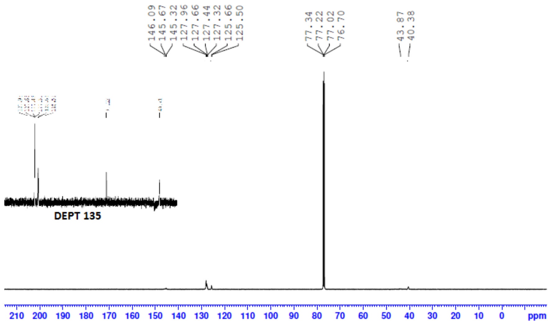
Figura 17. Espectro RMN ^{13}\text{C} e DEPT 135 do copolímero AI2, em \text{CDCl}_3
