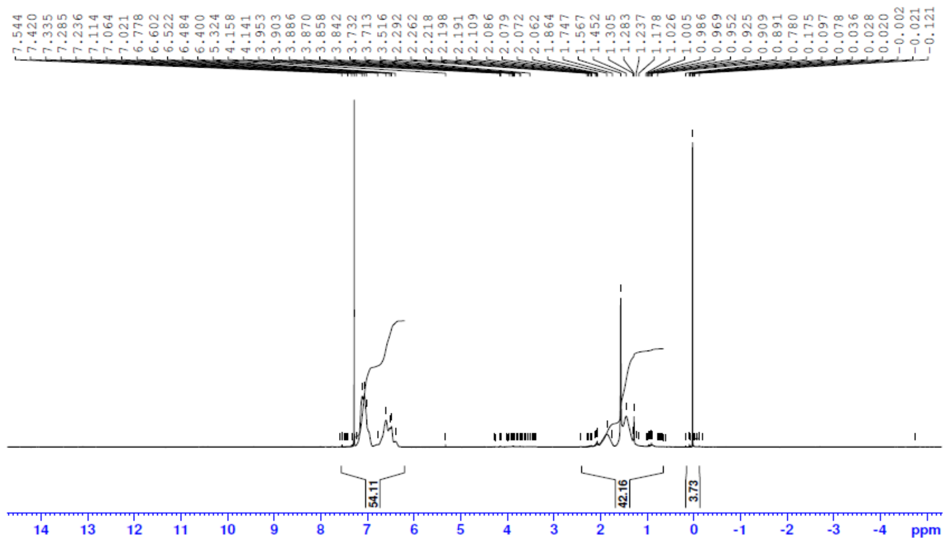
Figura 7. Espectro RMN ^1\text{H} do copolímero AA10, em \text{CDCl}_3
