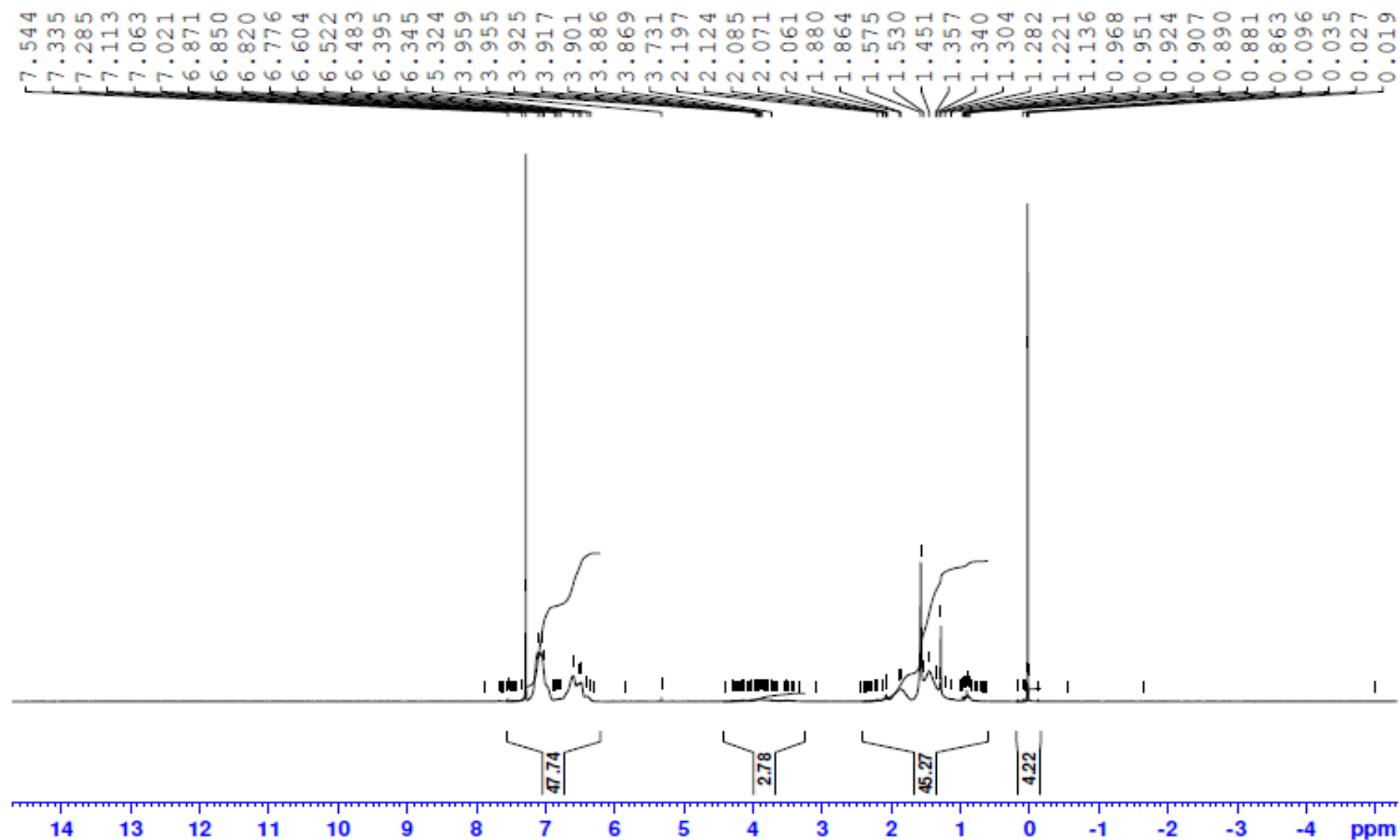
Figura 13. Espectro RMN ^1\text{H} do copolímero AA50, em \text{CDCl}_3
