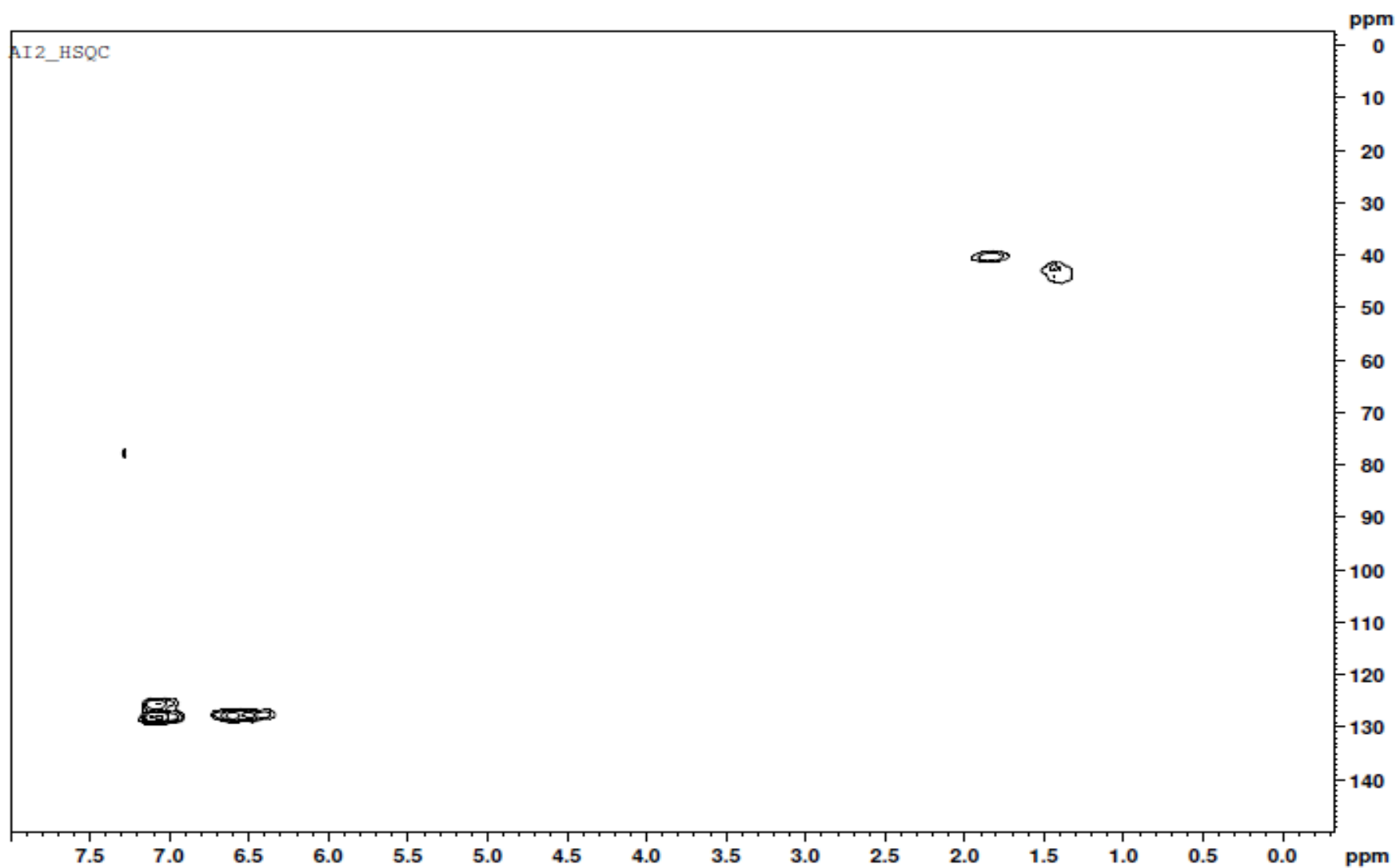
Figura 18. Espectro RMN HSQC do copolímero AI2, em \text{CDCl}_3
