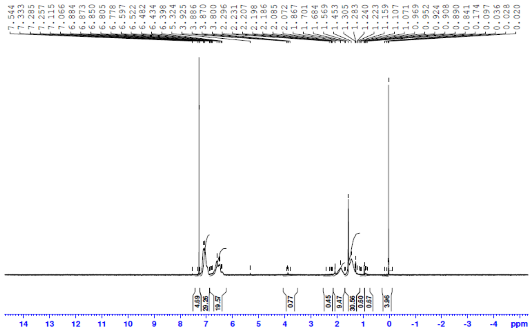
Figura 10. Espectro RMN ^1\text{H} do copolímero AA20, em \text{CDCl}_3
