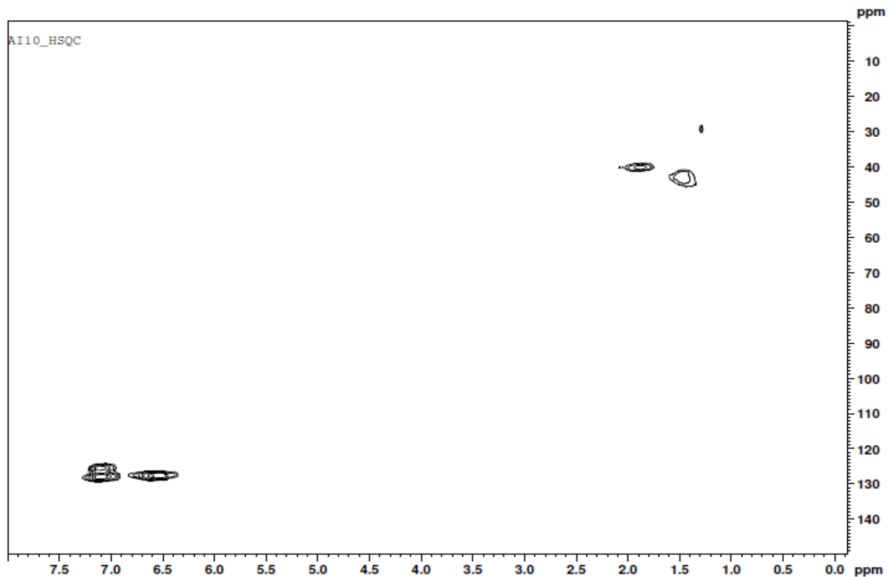
Figura 24. Espectro RMN HSQC do copolímero AI10, em \text{CDCl}_3
