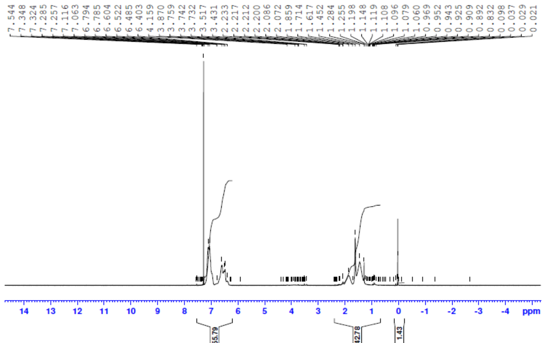
Figura 19. Espectro RMN ^1\text{H} do copolímero Al5, em \text{CDCl}_3
