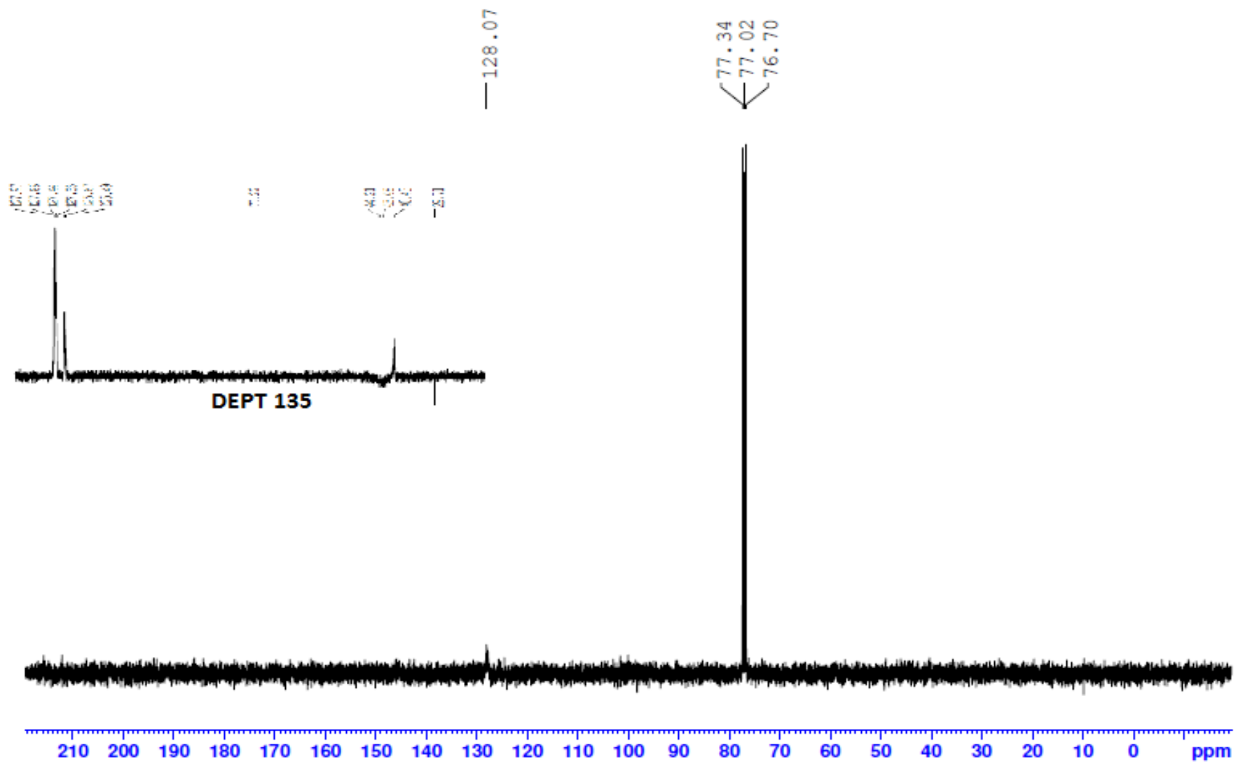
Figura 25. Espectro RMN 13 C e DEPT 135 do copolímero AI20, em CDCl 3
