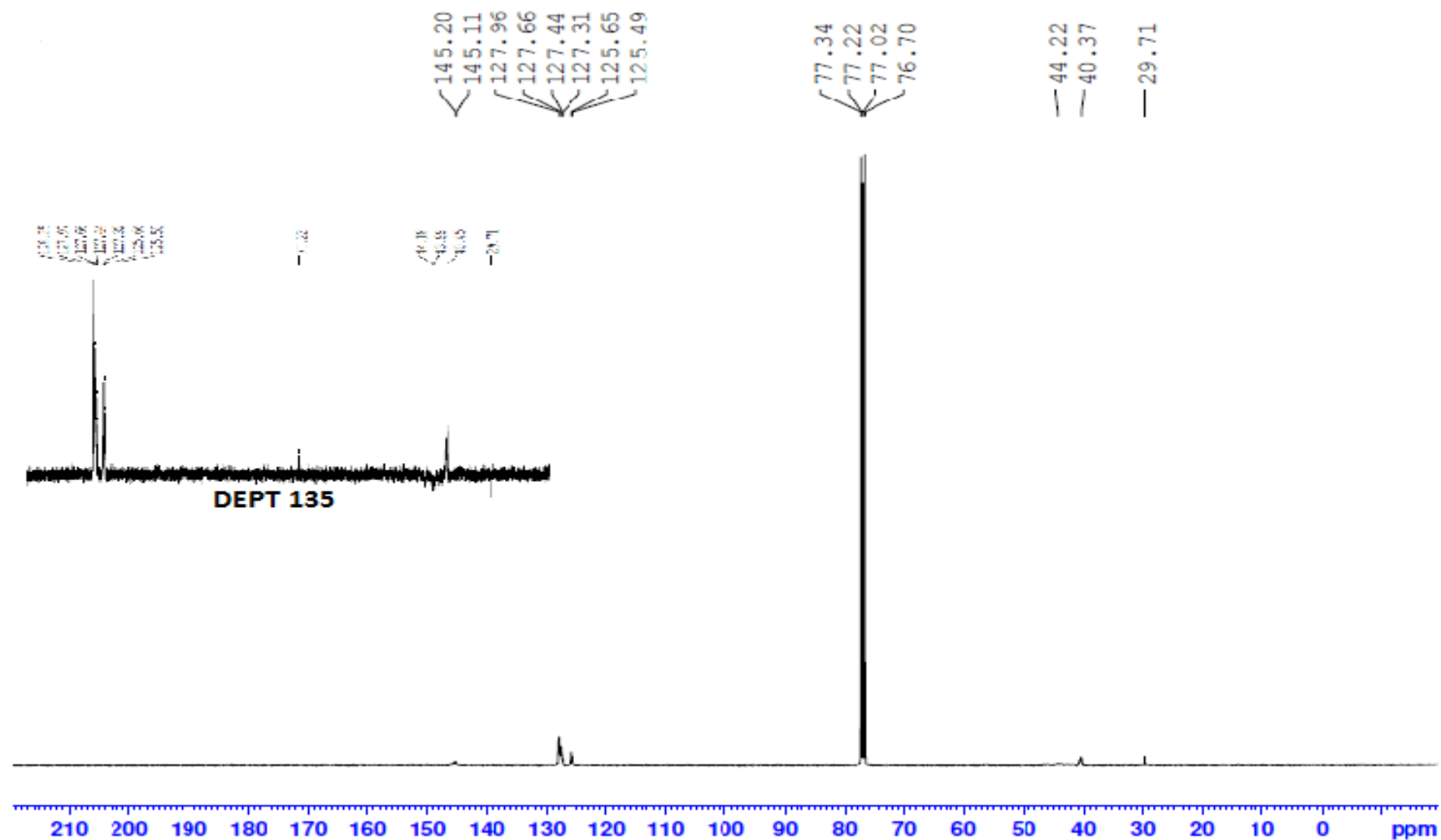
Figura 27. Espectro RMN ^{13}\text{C} e DEPT 135 do copolímero AI50, em \text{CDCl}_3
