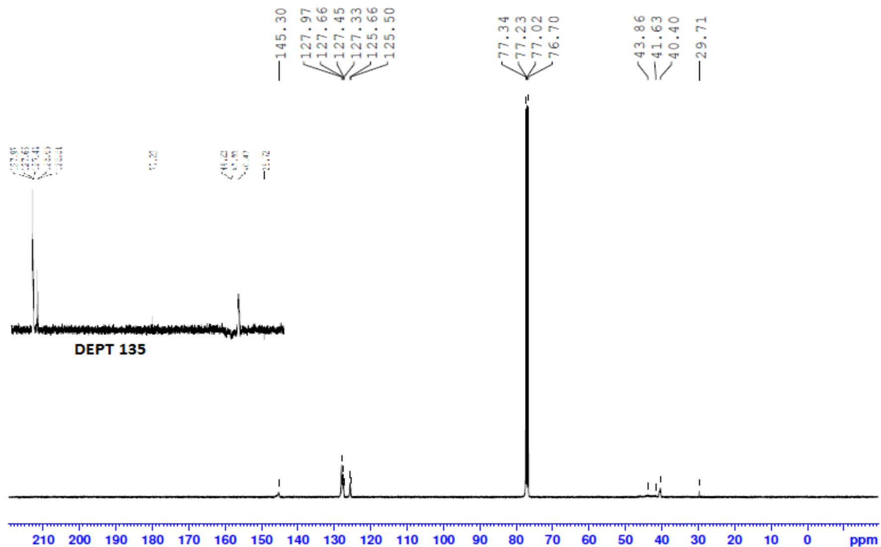
Figura 23. Espectro RMN ^{13}\text{C} e DEPT 135 do copolímero AI10, em \text{CDCl}_3
