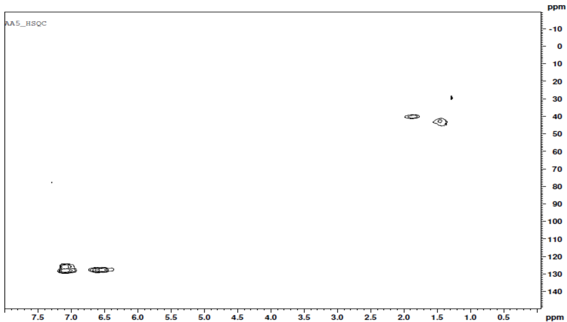
Figura 6. Espectro RMN HSQC do copolímero AA5, em \text{CDCl}_3
