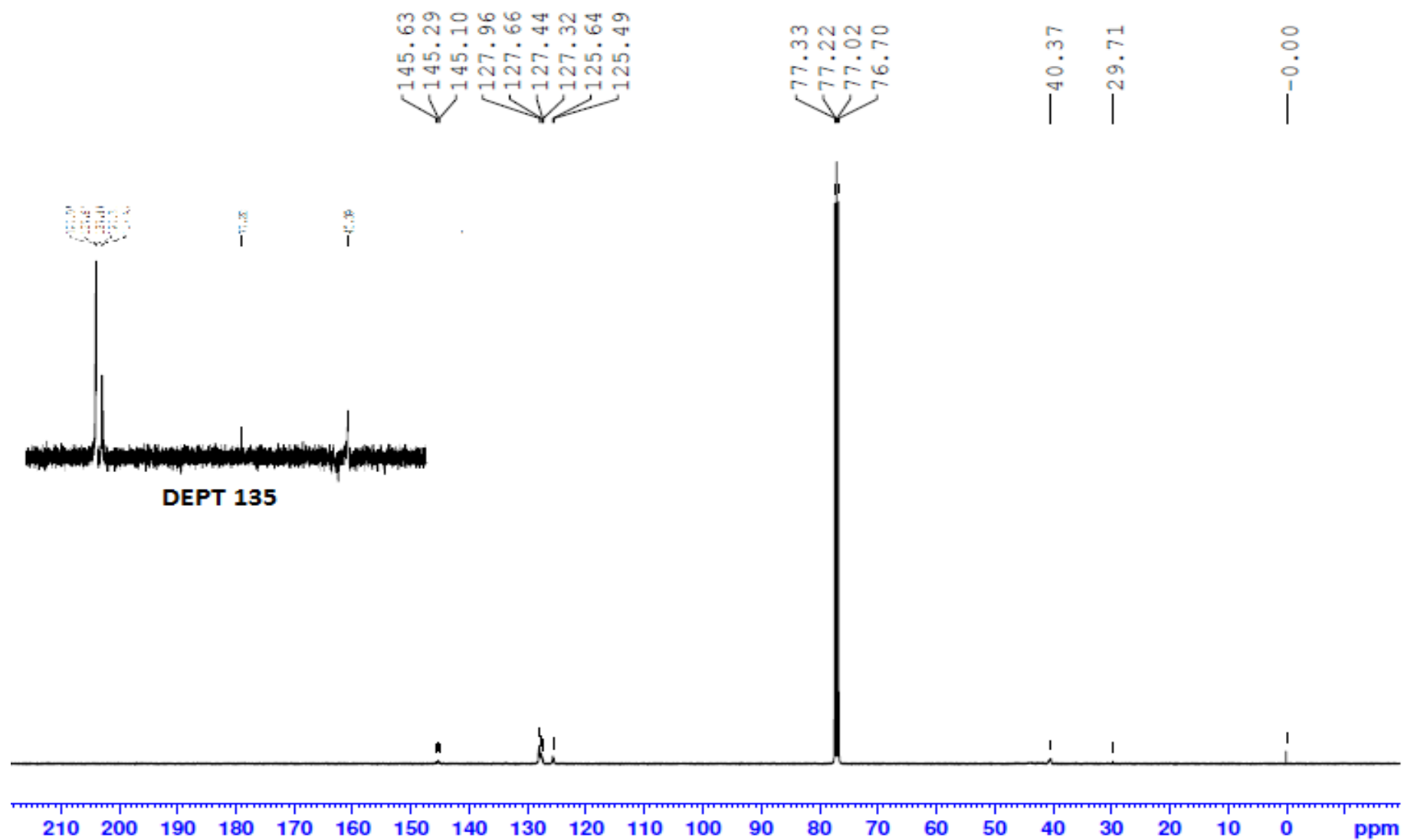
Figura 11. Espectro RMN ^{13}\text{C} e DEPT 135 do copolímero AA20, em \text{CDCl}_3
