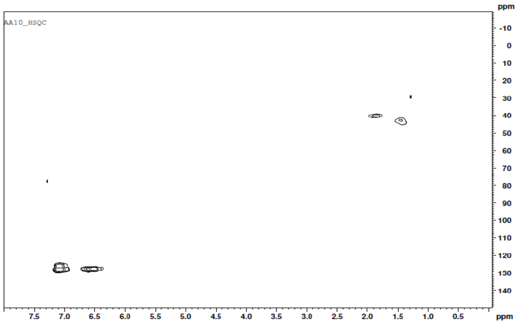
Figura 9. Espectro RMN HSQC do copolímero AA10, em \text{CDCl}_3
