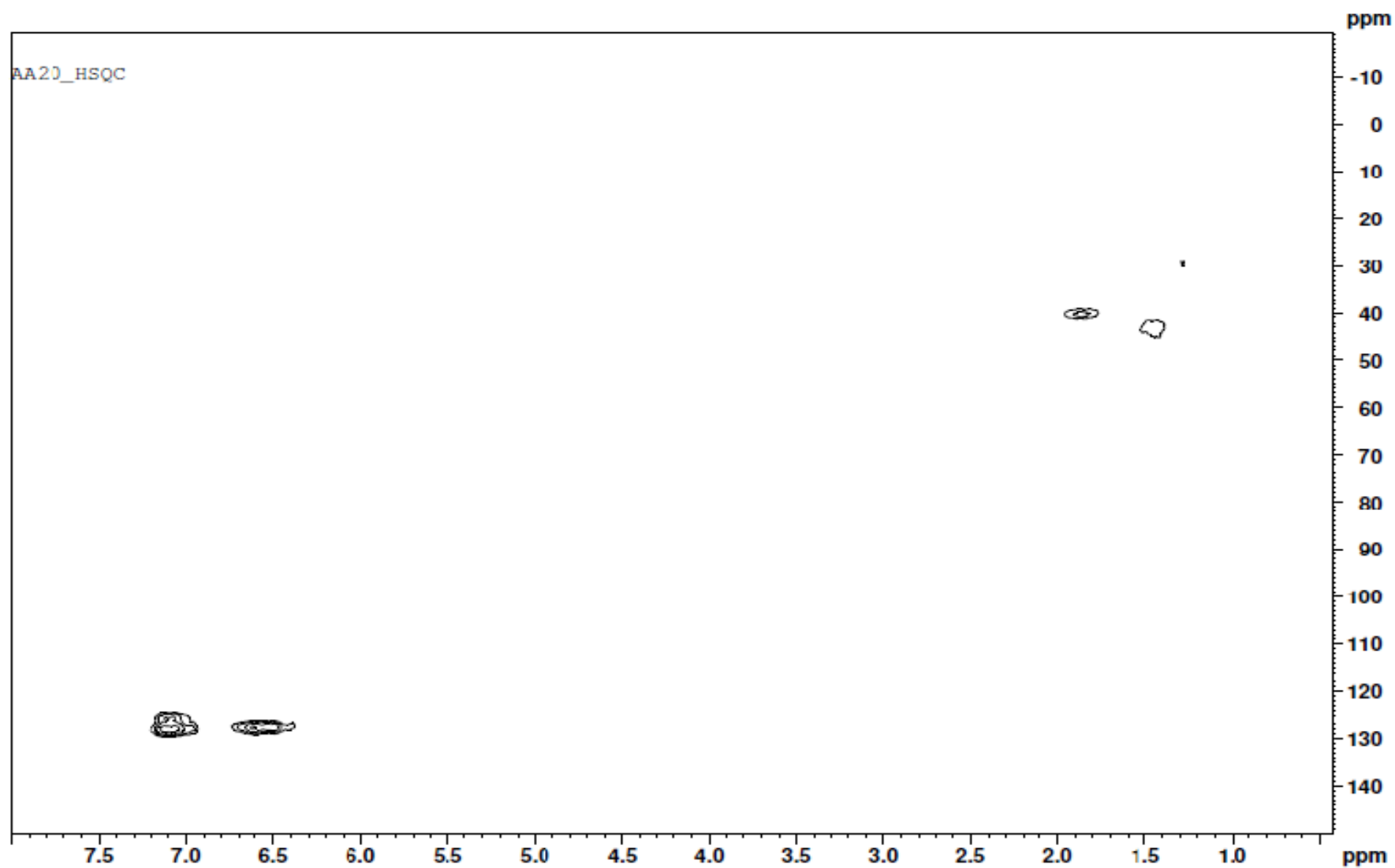
Figura 12. Espectro RMN HSQC do copolímero AA20, em \text{CDCl}_3
