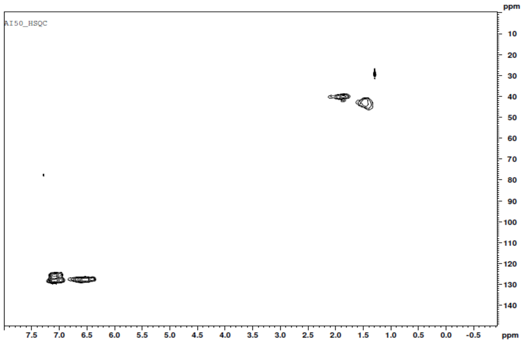
Figura 28. Espectro RMN HSQC do copolímero AI50, em \text{CDCl}_3
