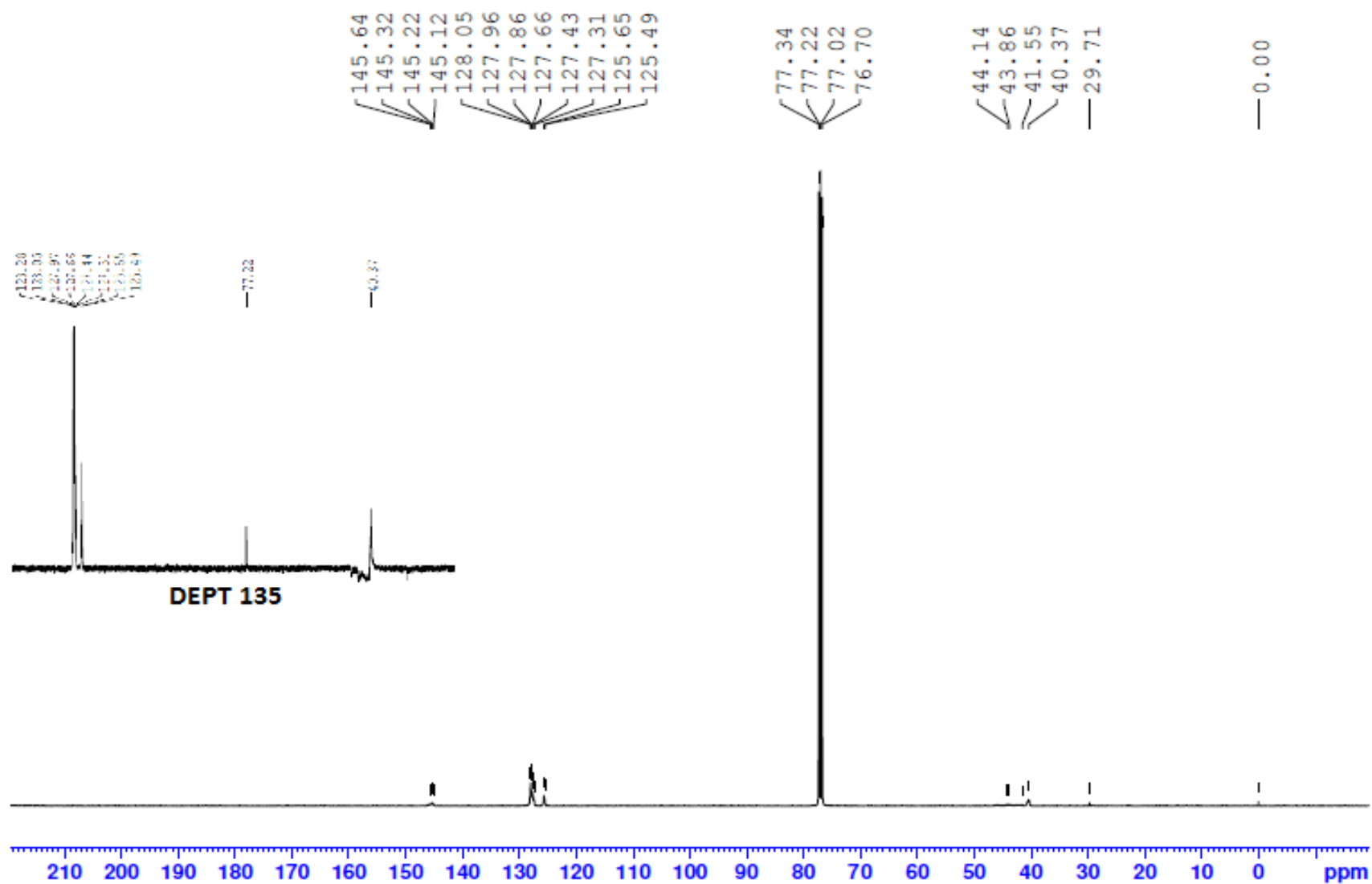
Figura 20. Espectro RMN 13 C e DEPT 135 do copolímero AI5, em CDCl 3
