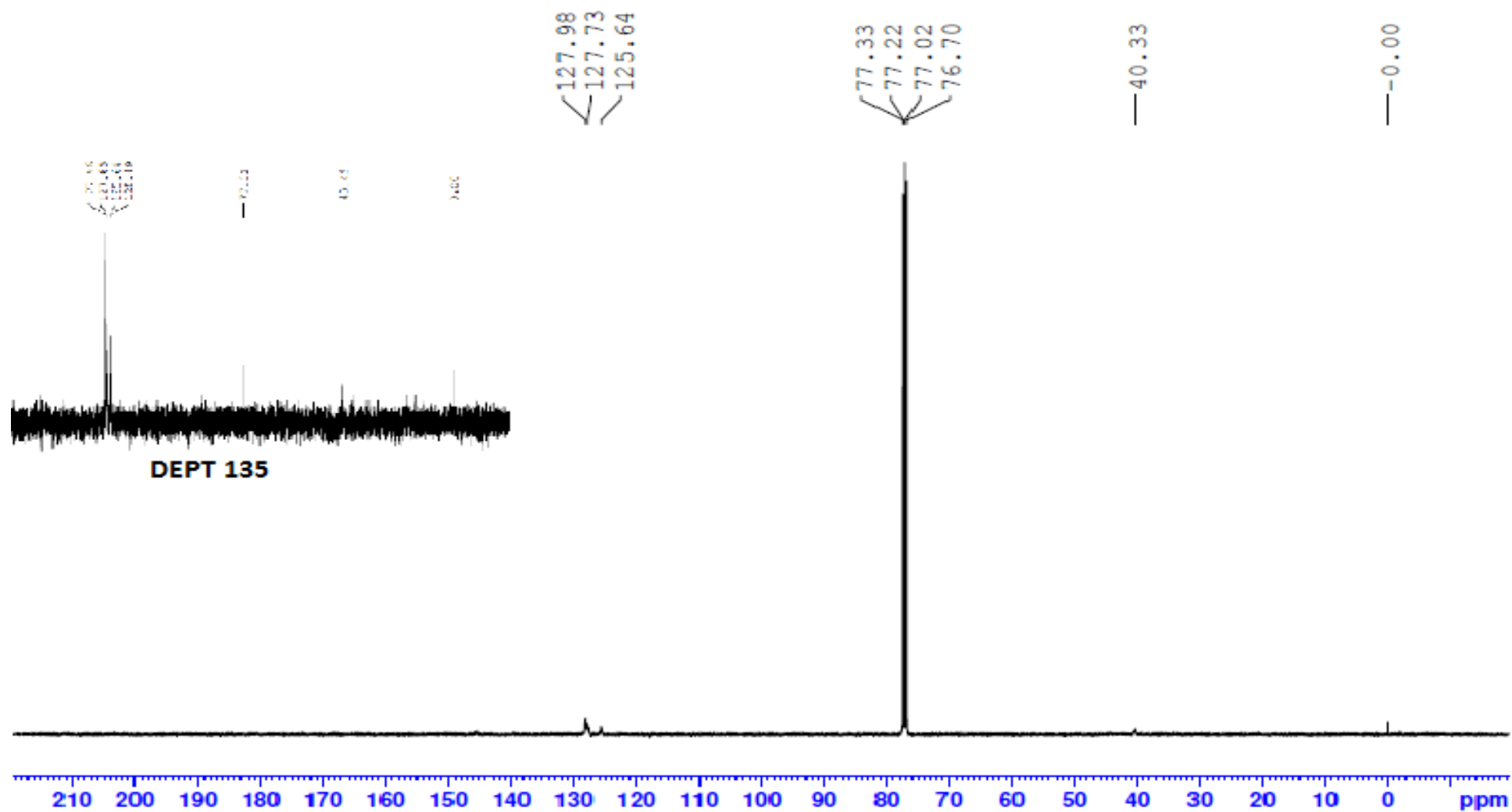
Figura 2. Espectro de RMN ^{13}\text{C} e DEPT 135 do copolímero AA2, em \text{CDCl}_3
