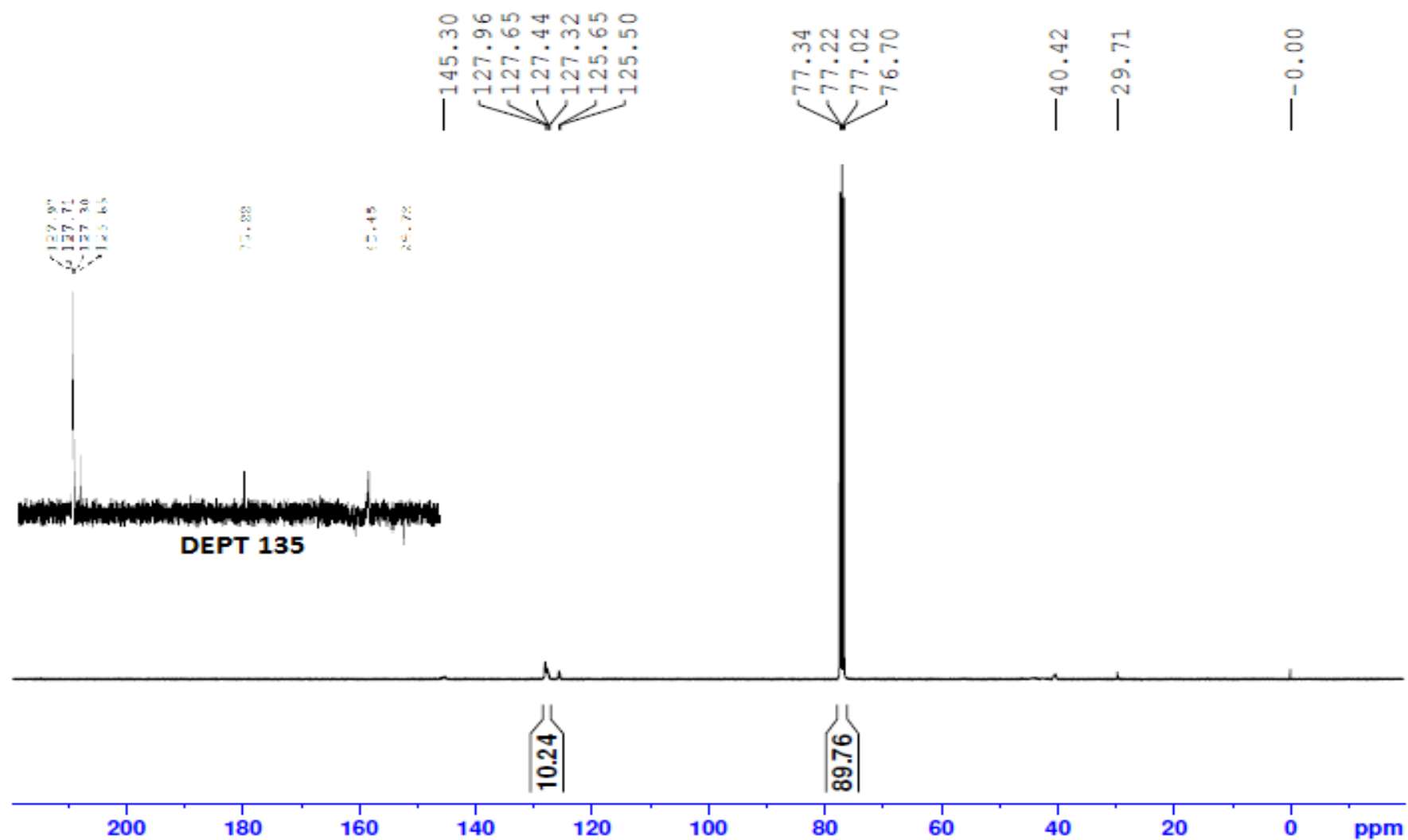
Figura 14. Espectro RMN ^{13}\text{C} e DEPT 135 do copolímero AA50, em \text{CDCl}_3
