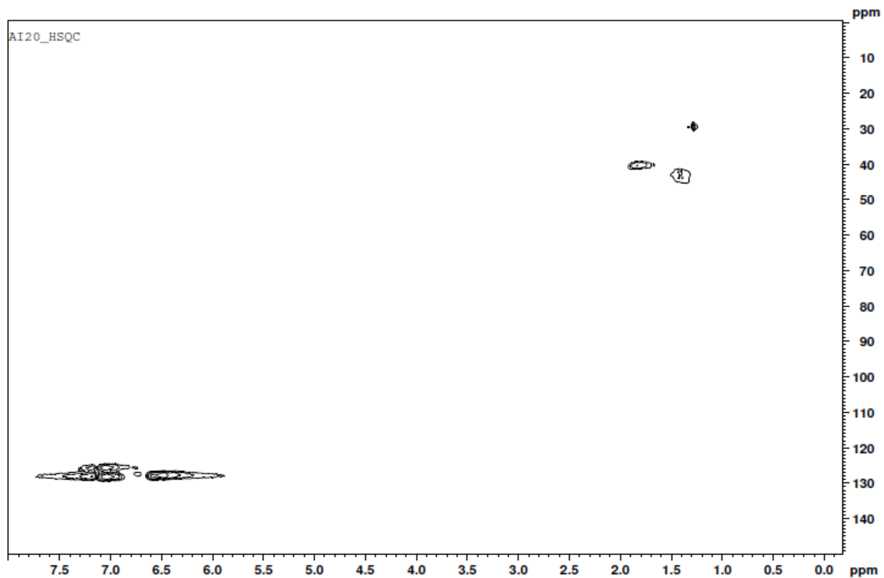
Figura 26. Espectro RMN HSQC do copolímero AI20, em CDCl 3
