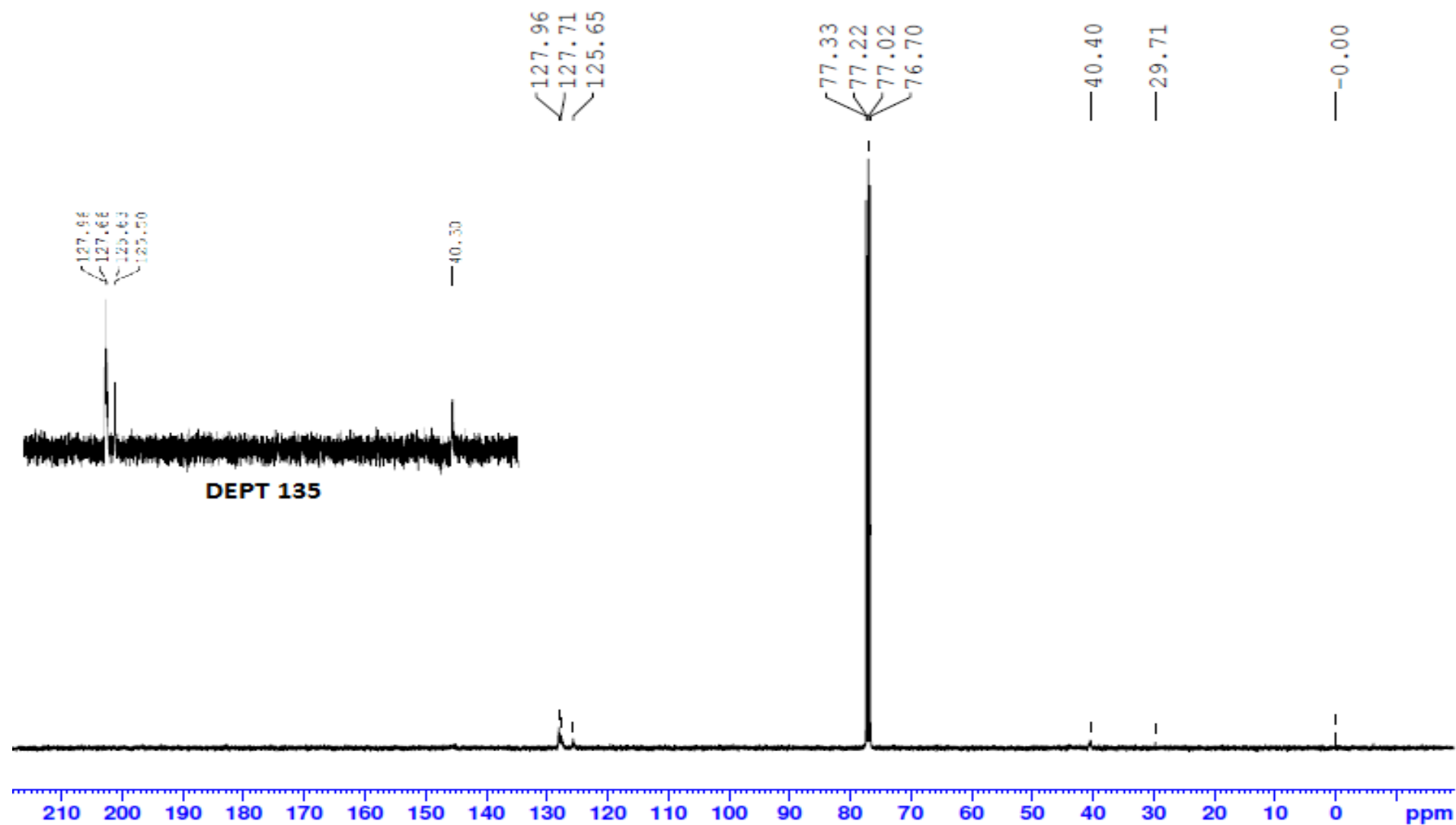
Figura 8. Espectro RMN ^{13}\text{C} e DEPT 135 do copolímero AA10, em \text{CDCl}_3
