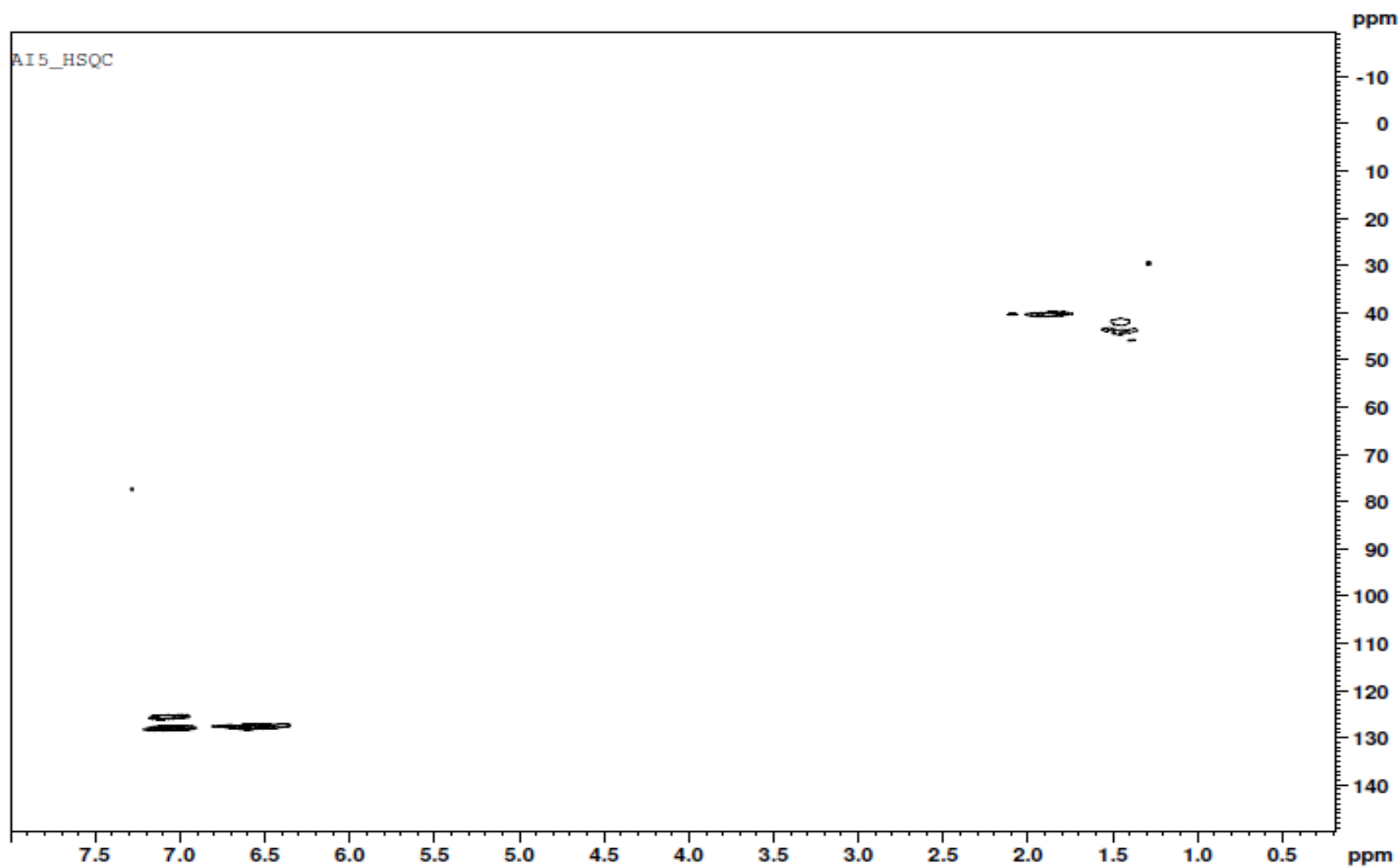
Figura 21. Espectro RMN HSQC do copolímero AI5, em \text{CDCl}_3
