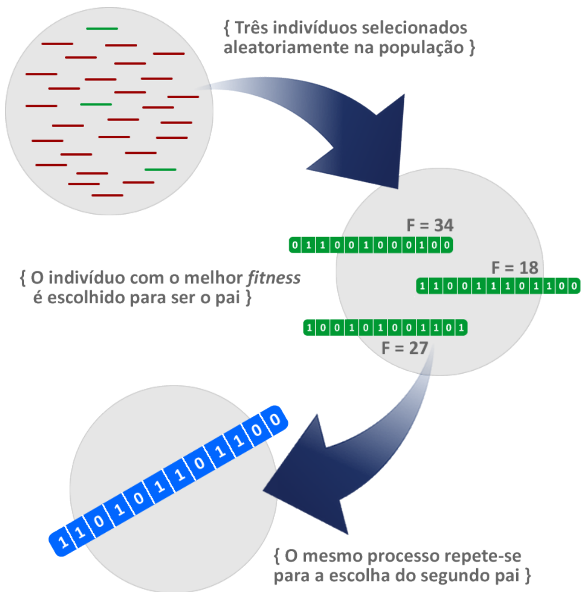
Figura 8: Processo de Seleção por Torneio
