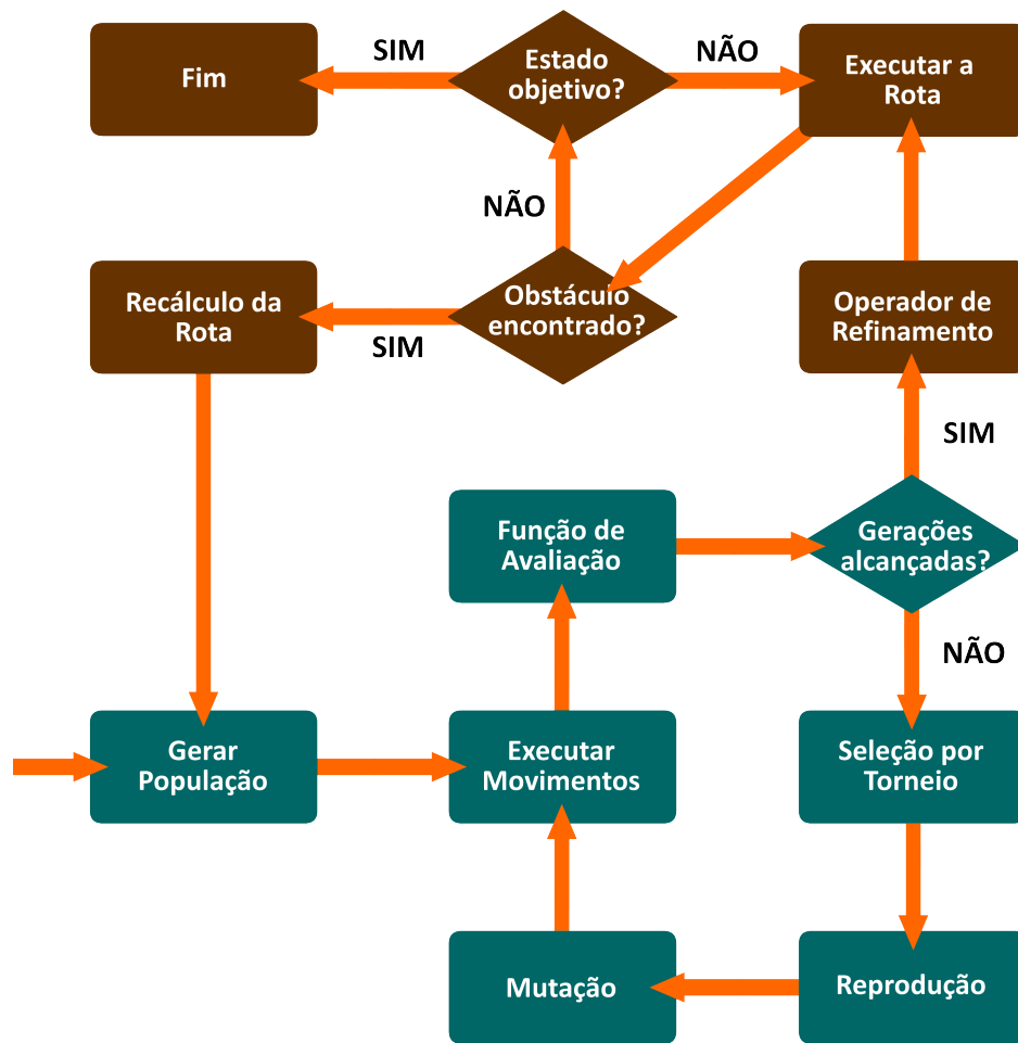
Figura 6: Fluxograma do Modelo Evolucionário de Planejamento de Rotas de Robôs
