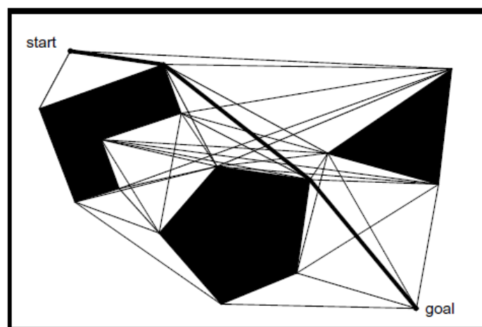
Figura 2: Abordagem Clássica de Roadmap: Grafo de Visibilidade
