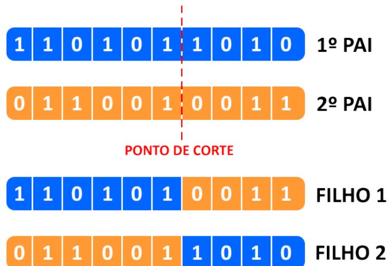
Figura 9: Operador de crossover de um ponto
