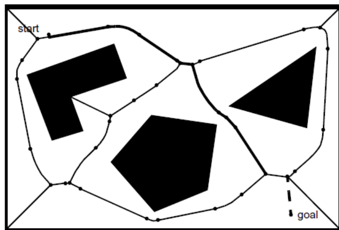
Figura 3: Abordagem Clássica de Roadmap: Diagrama de Voronoi
