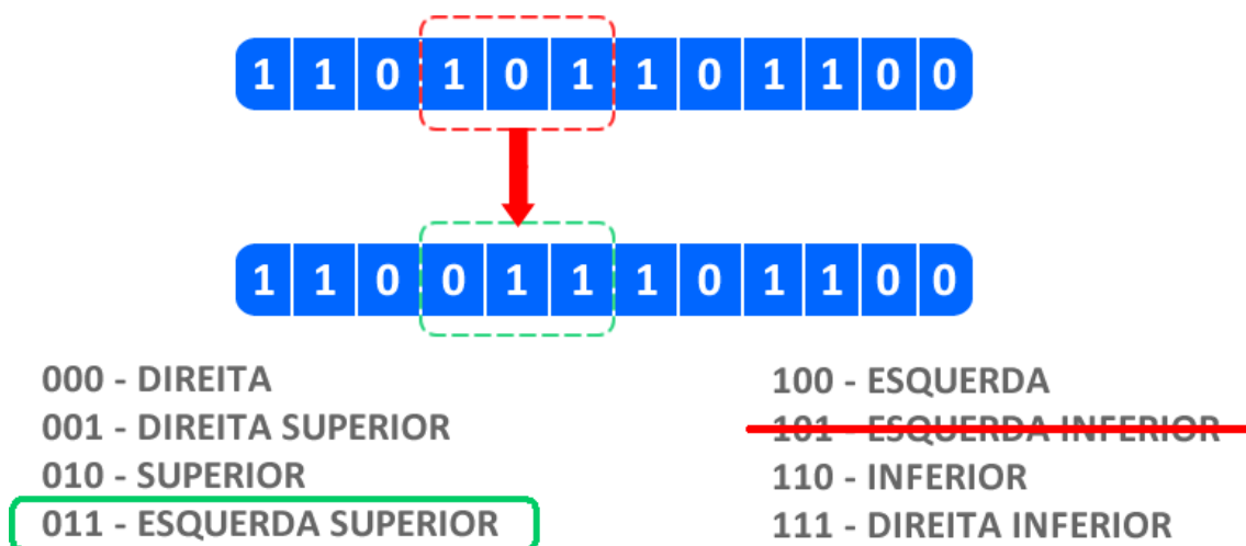
Figura 10: Operador de mutação atuando sobre um gene de um cromossomo
