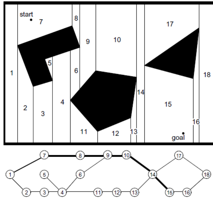
Figura 4: Abordagem Clássica de Decomposição de Células
