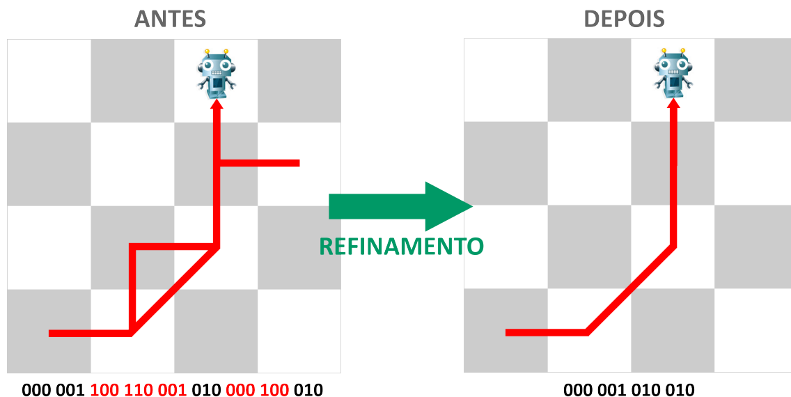
Figura 11: Otimização da rota através do operador de refinamento
