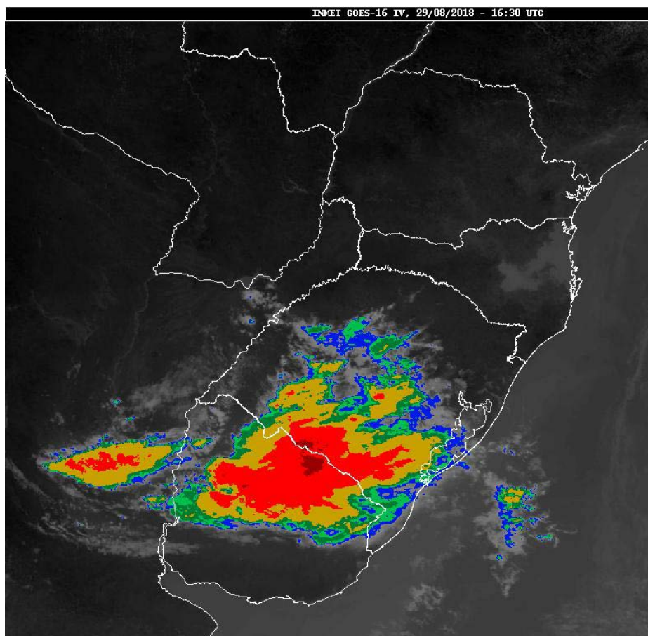
Figura 1. Imagem do satélite GOES 16, canal infravermelho, do dia 29/08/2018 às 13:30h (horário de Brasília). Fonte da imagem: Instituto Nacional de Meteorologia (INMET).
