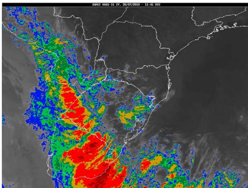
Figura 1. Imagem do satélite GOES 16, canal infravermelho, do dia 20/07/2018 às 8h45m (horário de Brasília).
